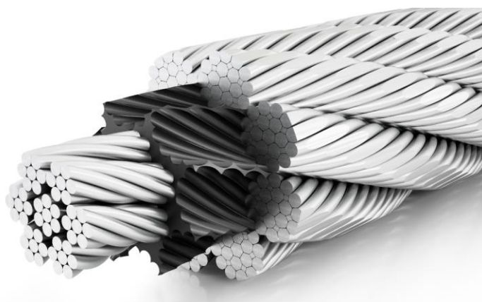
Lina 8-splotkowa PYTHON z technologią PlastGuard®
