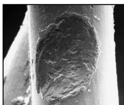
Uszkodzenie drutu pod mikroskopem spowodowane naciskiem punktowym
